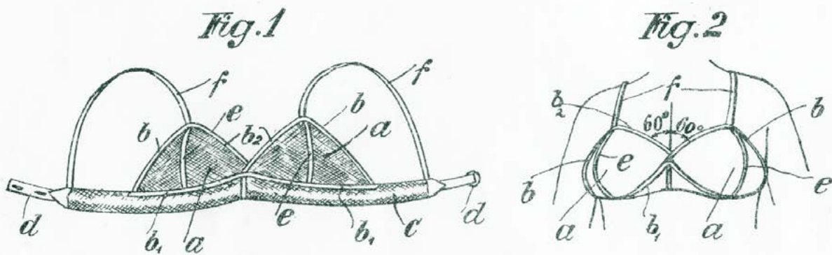
Konstruktionszeichnung des 1932 von Eugenie Thöny zum Patent angemeldeten Büstenhalters | Original: Wirtschaftsarchiv Vorarlberg, Bestand Patentschriften, Sig. A/2995
