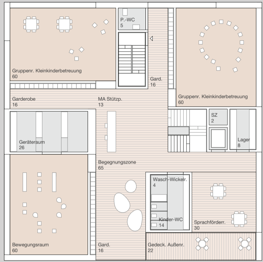
E+1 | Kinderhaus | Kleinkindergruppen | Bewegungsraum 1.200
