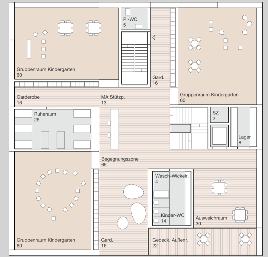
E+2 u. E+3 | Kinderhaus | Gruppenraum 1.200
