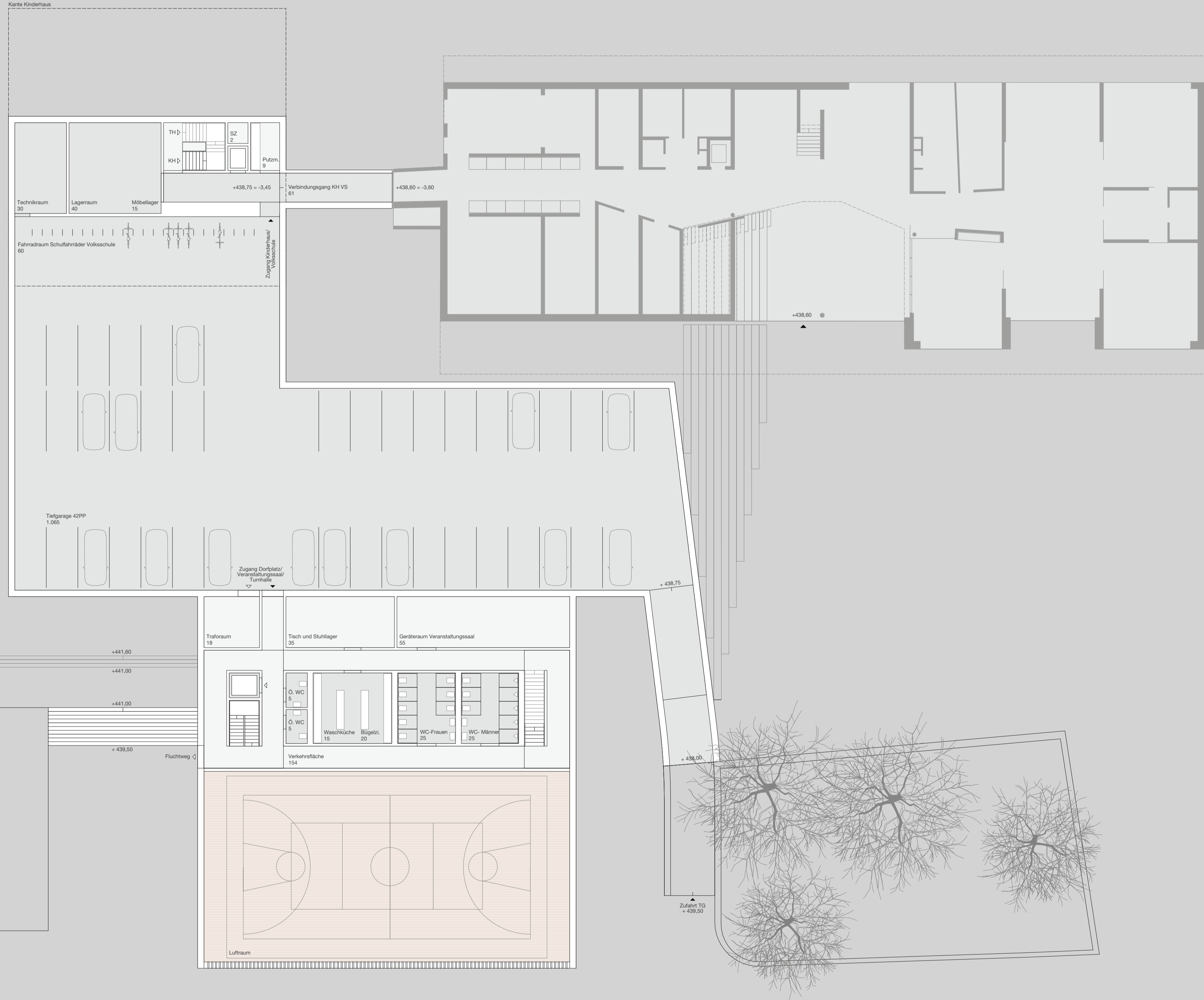
E-1 | Turn- und Veranstaltungshaus | Tiefgarage 1.200
