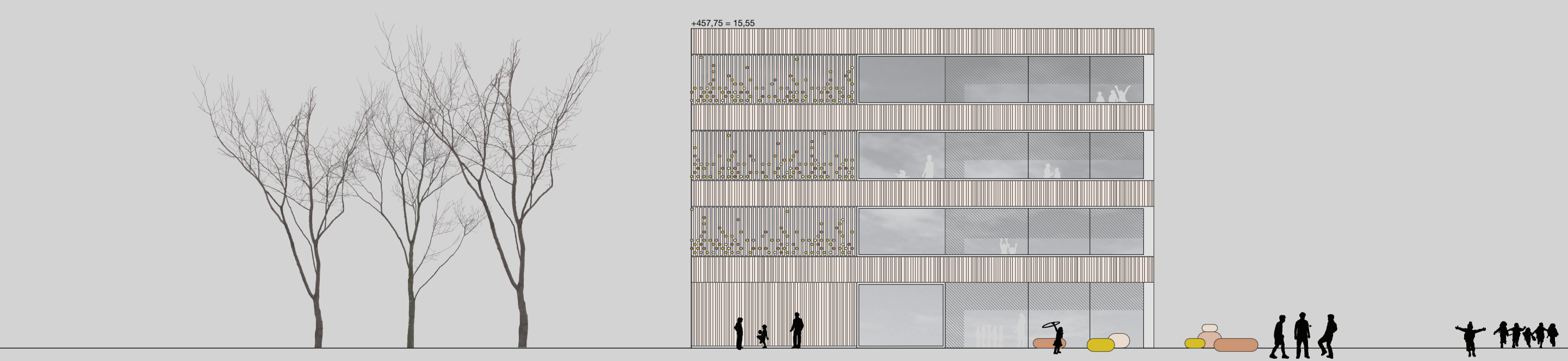
Westfassade | Kinderhaus 1:200
